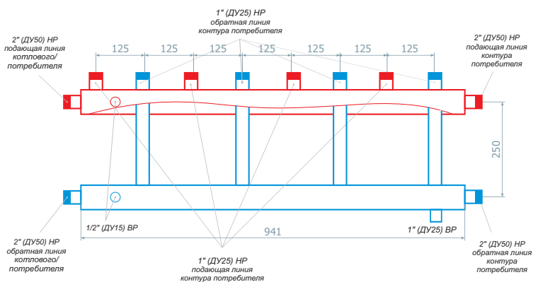
КМГ250-4Вх25
