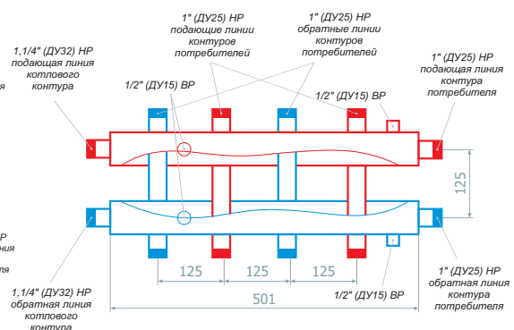
КМГ60-5BY
