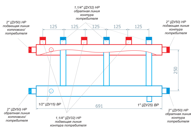
КМГ250-3Вх32
