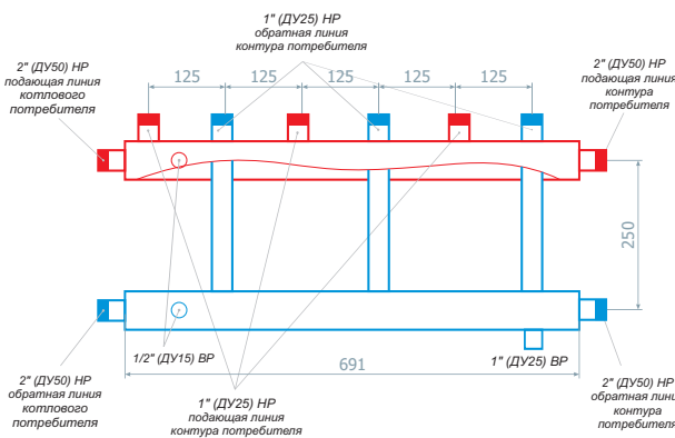
КМГ250-3Вх25
