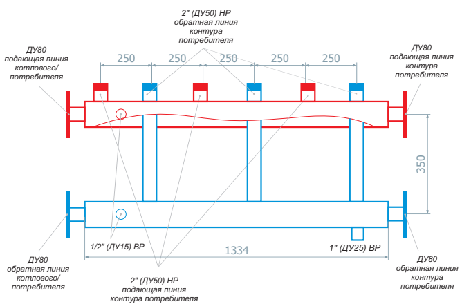
КМГ(Ф)600-3Вх50
