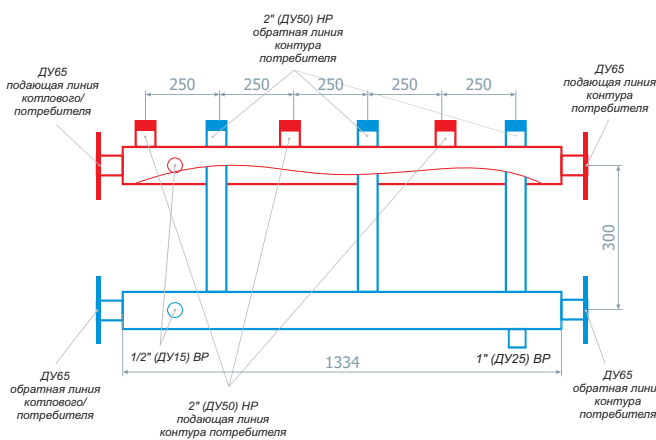
КМГ(Ф)400-3Вх50
