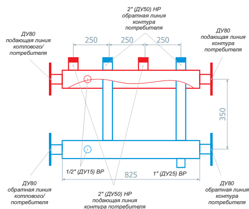
КМГ(Ф)600-2Вх50
