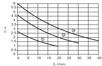
Рабочее поле для насоса CR-25/8
