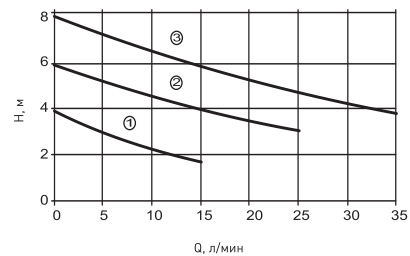
Рабочее поле для насоса CR-32/8
