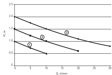
Рабочее поле для насосов CR-25/4 и CR-32/4
